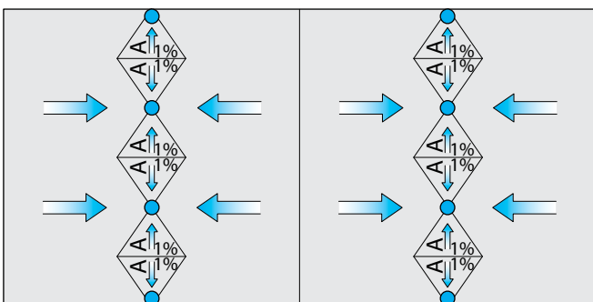
Abb. 11: Jeweils ein zweiseitiges Gefälle von 1,5% zu den Dachwassereinträufen, z.B. bei Metall- oder Holzunterkonstruktionen, mit einer aufgesetzten Gefälledämmung (A) zwischen den Einläufen. Dachwassereinträge an die sanitären Entwässerungsleitungen angeschlossen.
