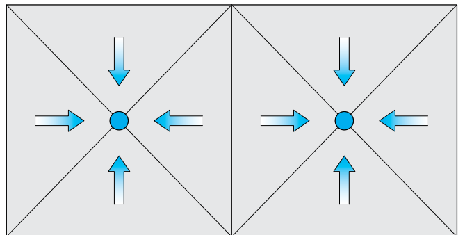
Abb. 13: Allseitiges gleichmässiges Gefälle von 1,5%, Dachwassereinträge an die sanitären Entwässerungsleitungen angeschlossen.
