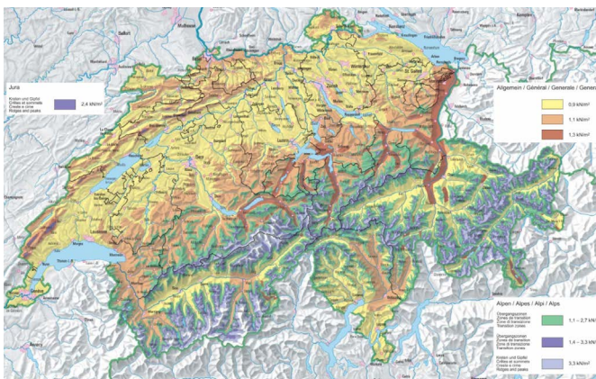
Abb. 3: Staudruckkarte «Einwirkungen auf Tragwerke» Staudruck (Anhang E) Auszug aus der Norm SIA 261
