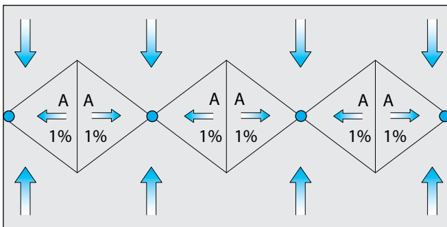
Abb. 10: Zweiseitiges Gefälle von 1,5% in die Mitte, zwischen den Einläufen eine aufgesetzte Gefälledämmung (A), Dachwassereinträge an die sanitären Entwässerungsleitungen angeschlossen.
